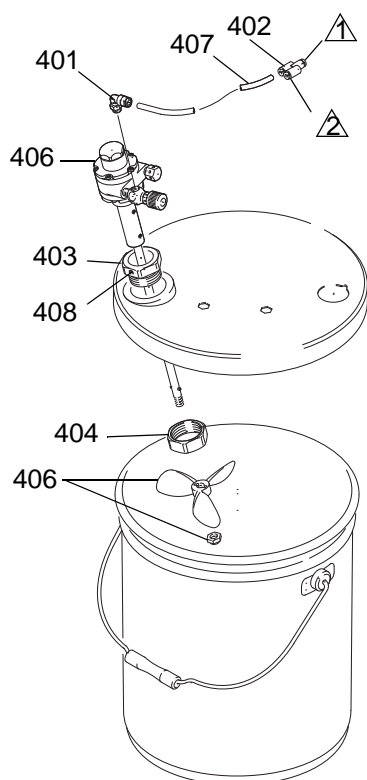
FIG. 13 245895 Agitator Kit
