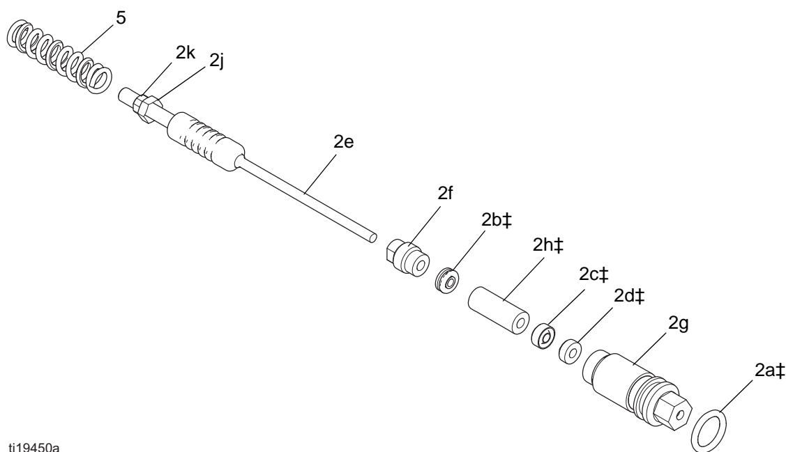
FIG. 31 . Packing Rod
