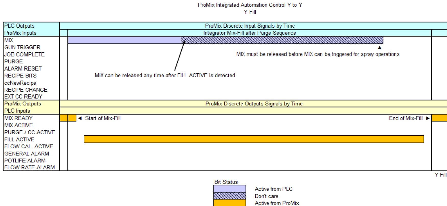
FIG. 80. Integration Control Y Fill
