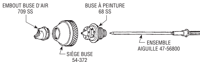
TABEAU DE SÉLECTION DE BUSES
